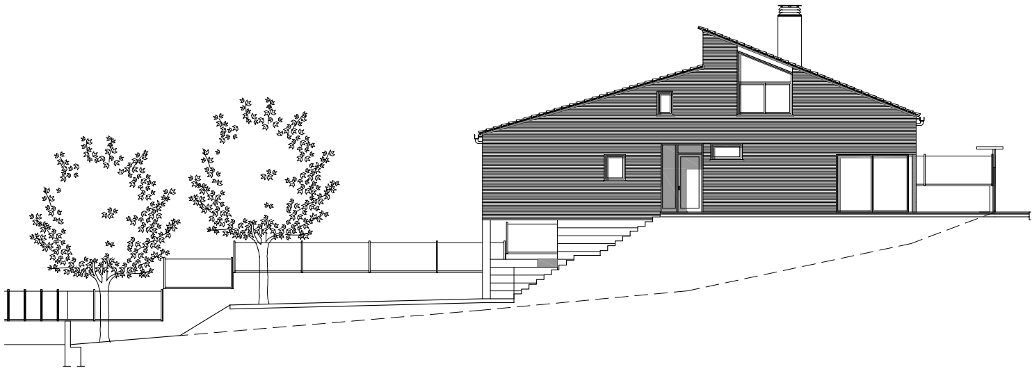
Façana Oest
