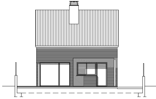
Façana Sud
