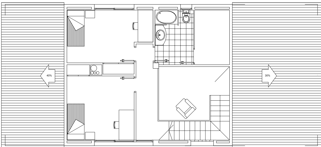
Planta primera
