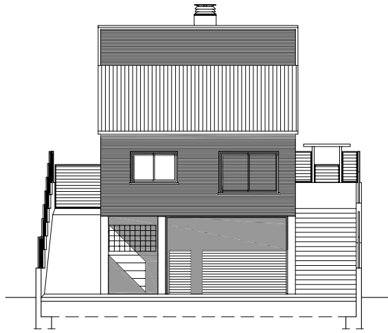
Façana Nord
