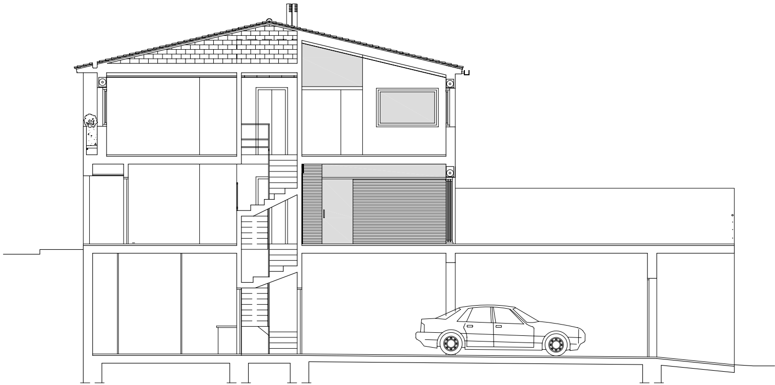
Secció
