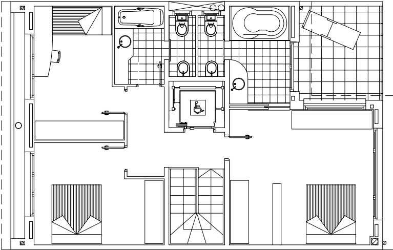
Planta primera
