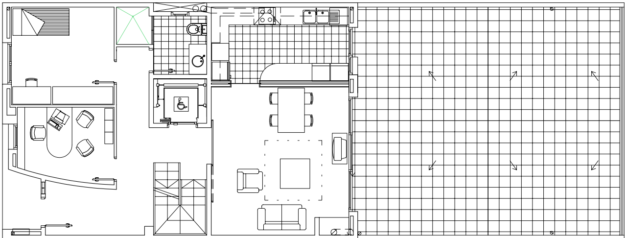
Planta baixa
