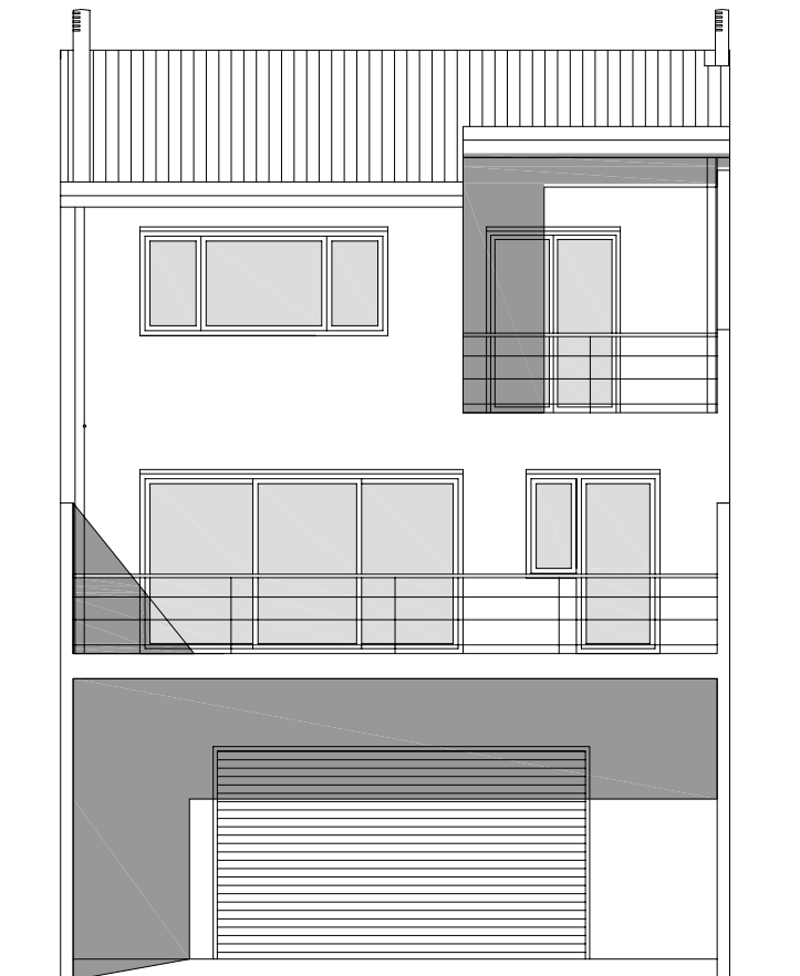
Façana Posterior
