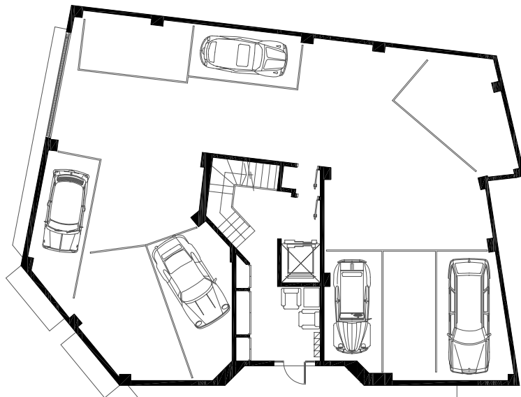
PLANTA BAIXA
