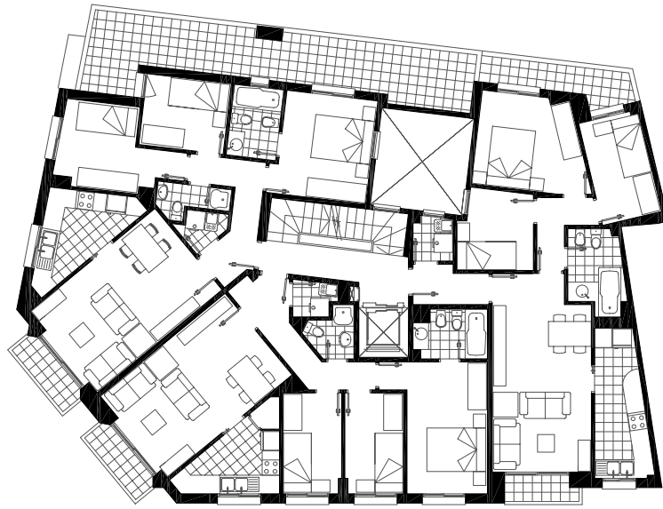
PLANTA TERCERA
