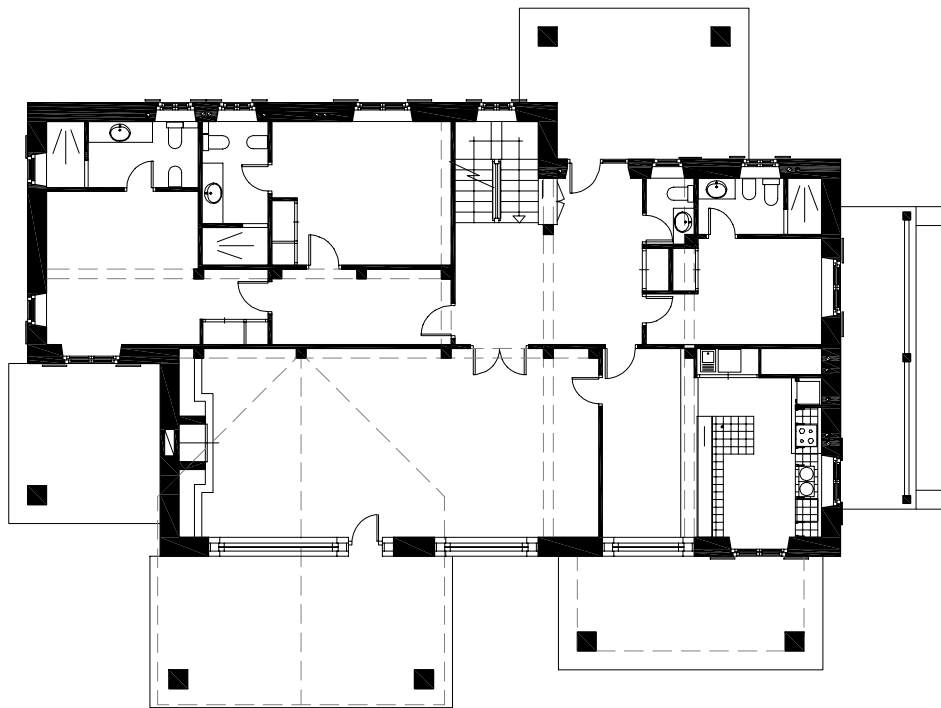
Planta baixa
