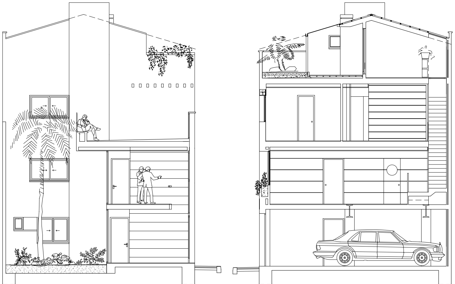
Seccions
