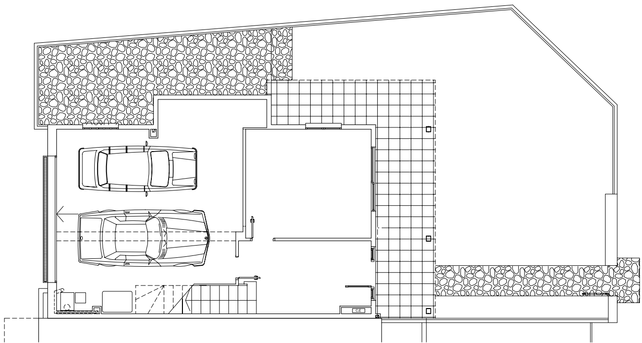
Planta baixa
