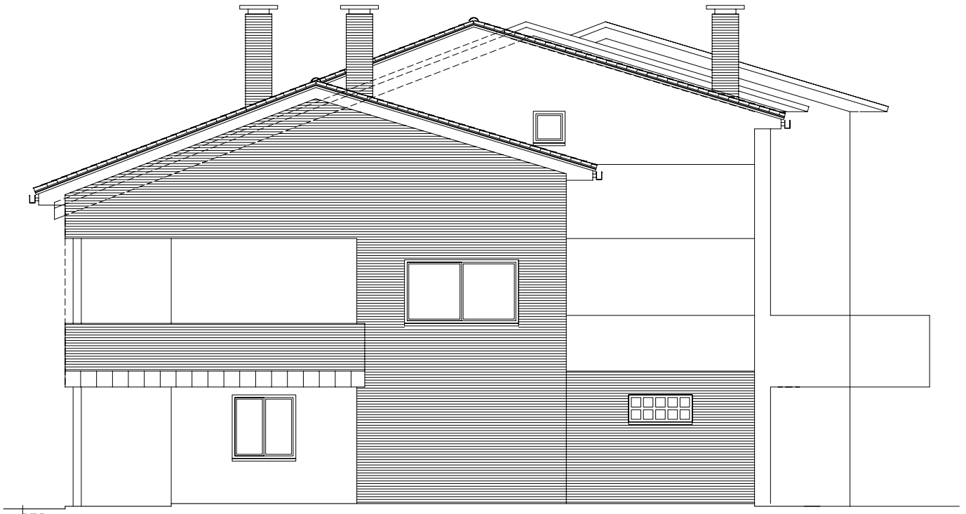
Façanes Sud
