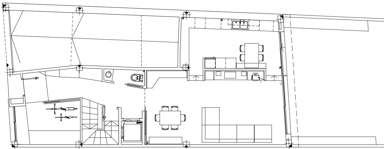
Planta baixa
